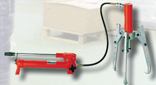
Hydraulique 700 bars
